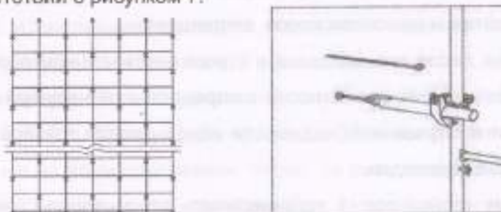
Рисунок 7 – Схема крепления лесов к стене.
